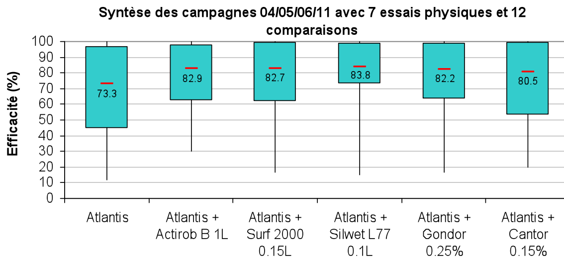
Figure 3 : Synthèse des campagnes 2004/2005/2006/2011, au sein de 7 essais sur vulpin ou ray grass, avec Atlantis WG associé ou non avec Actirob B, Surf 2000, Silwet L77, Gondor ou Cantor (12 comparaisons strictes).
