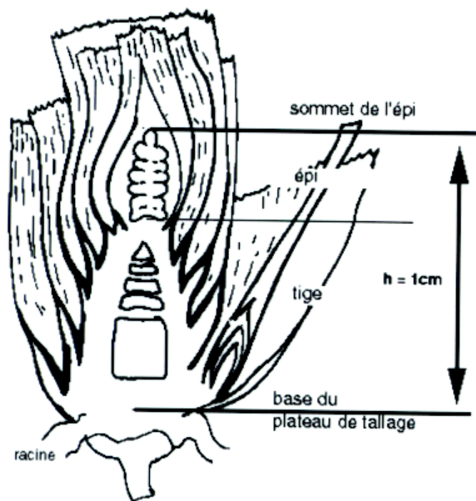
Figure 1 : Coupe de la base d'une plante à épi 1cm : le sommet de l'épi, différencié, est distant de la base du plateau de tallage de 10mm ; les entre-nœuds présents sous l'apex commencent à s'allonger (source : Gate, 1995).
